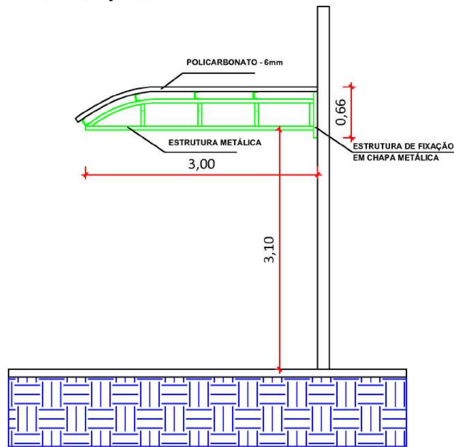
Corte sem o apoio da marquise
