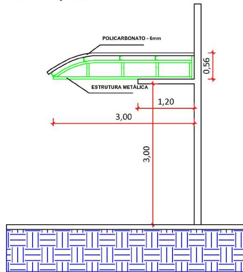
Corte com o apoio da marquise
